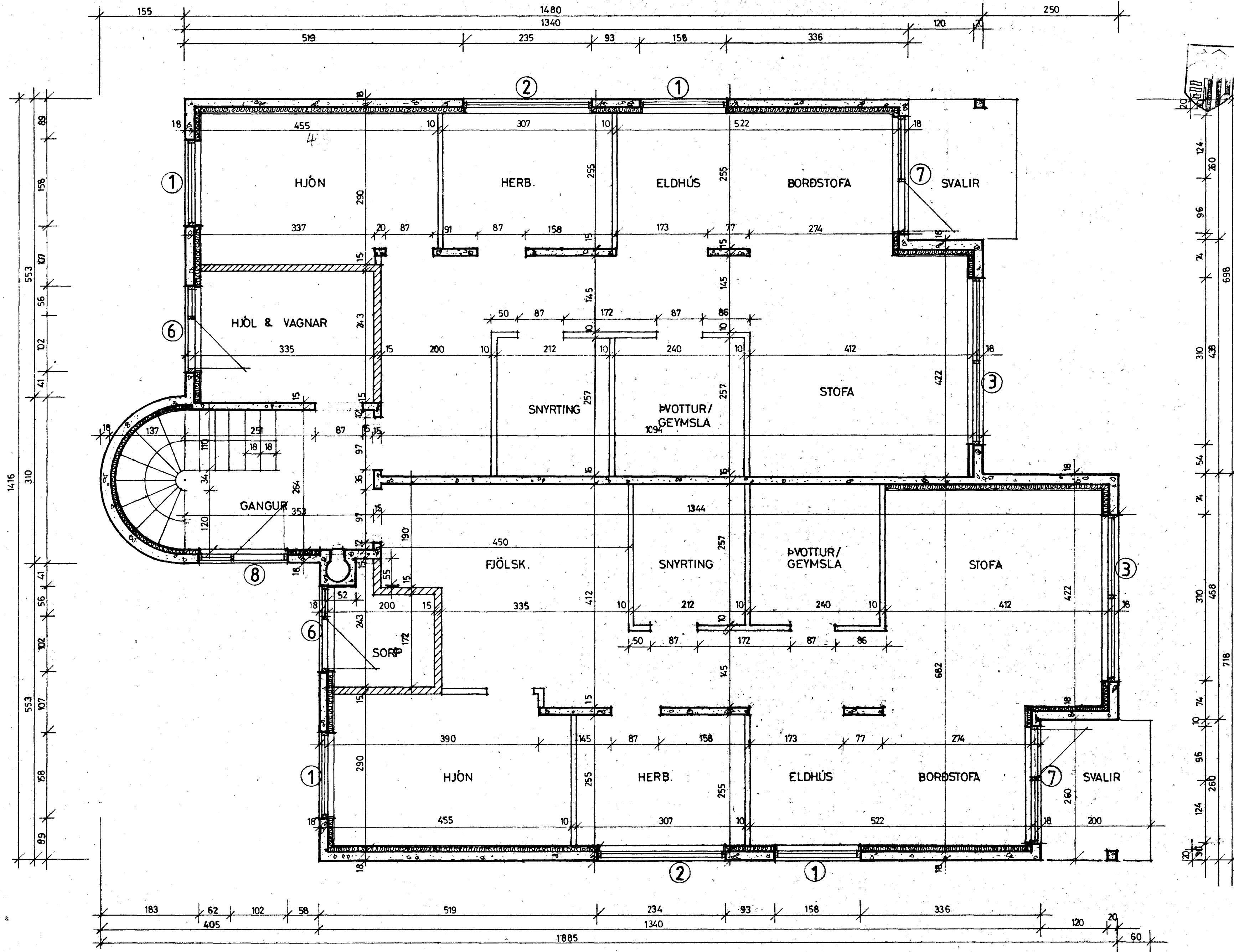
GRUNNMYND 1. HÆÐAR 1:50
