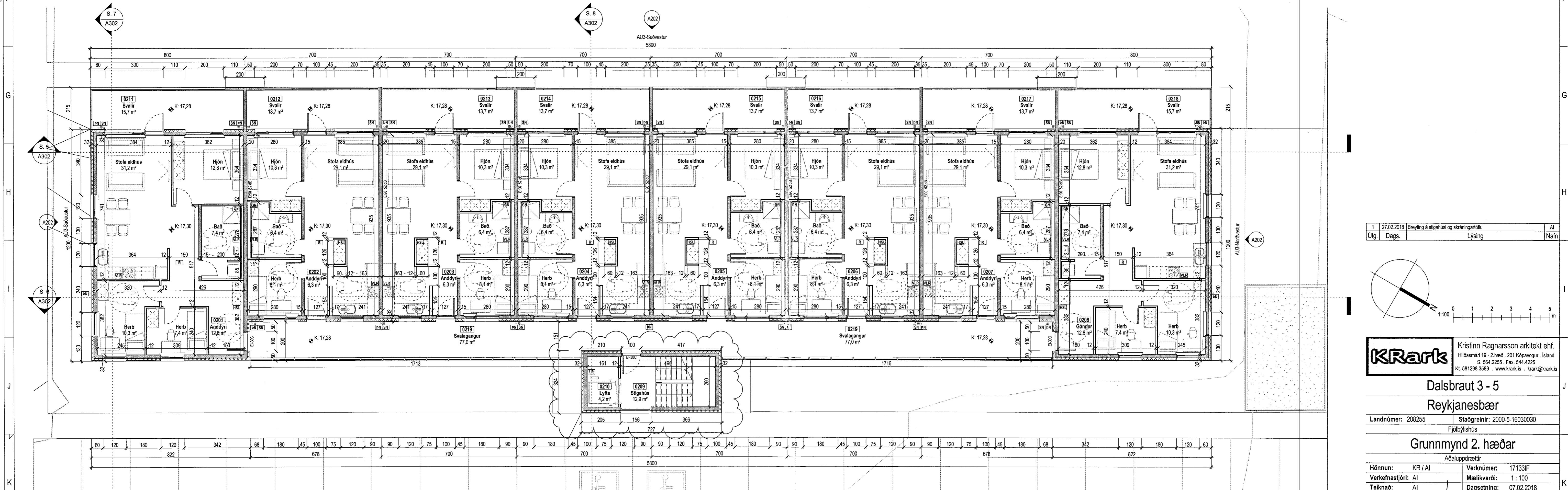
Grunnmynd 2. hæðar 1:100
